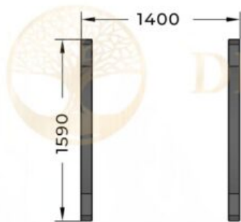
Sauna 1,6, Ø 200
